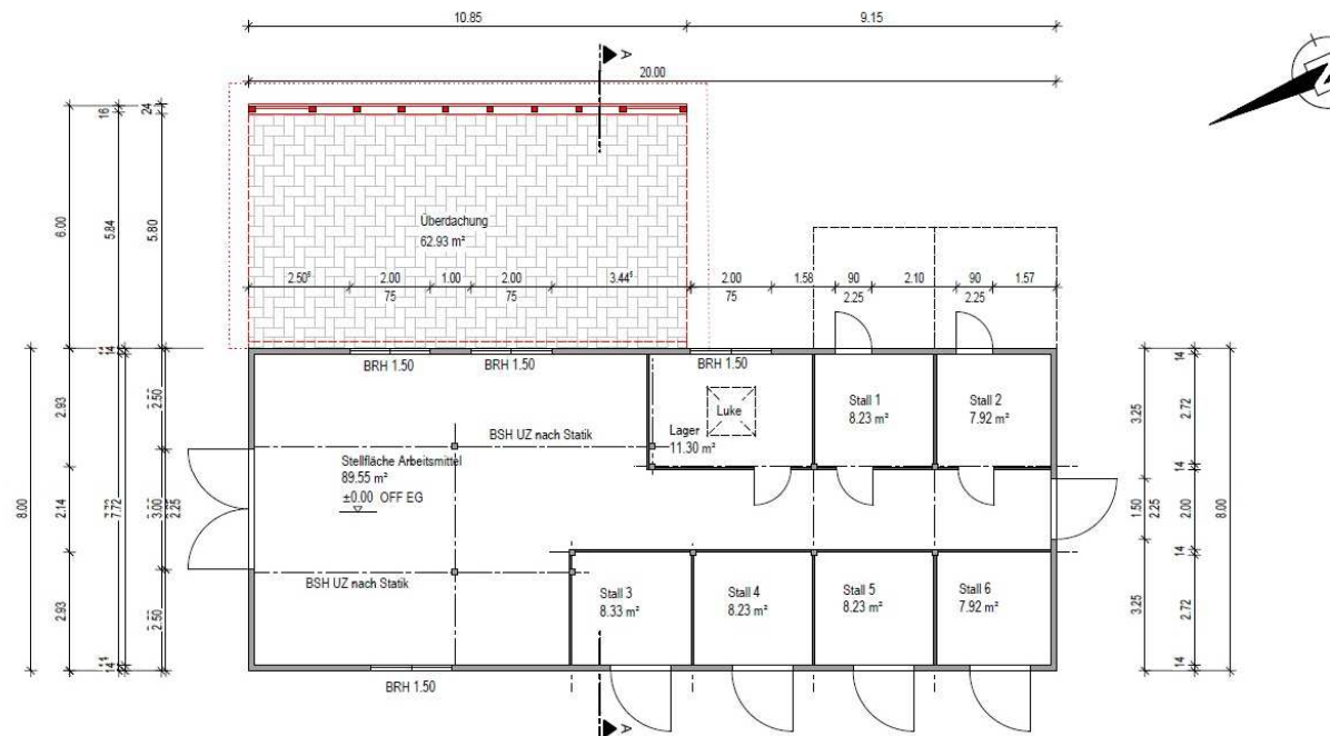
Grundriss Erdgeschoss M 1:100
