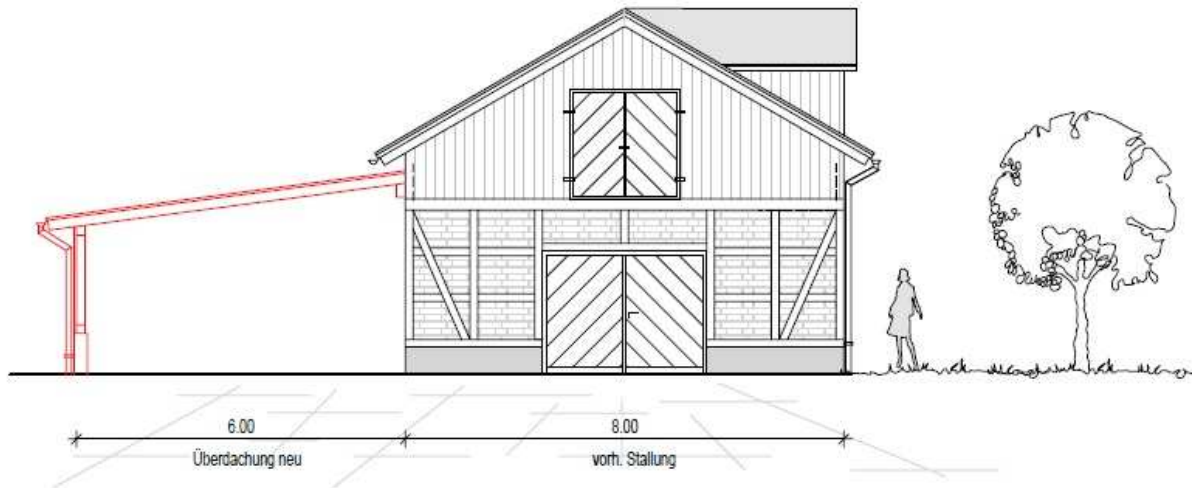
Nord-Ansicht
