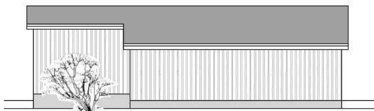
Nord - Ansicht
