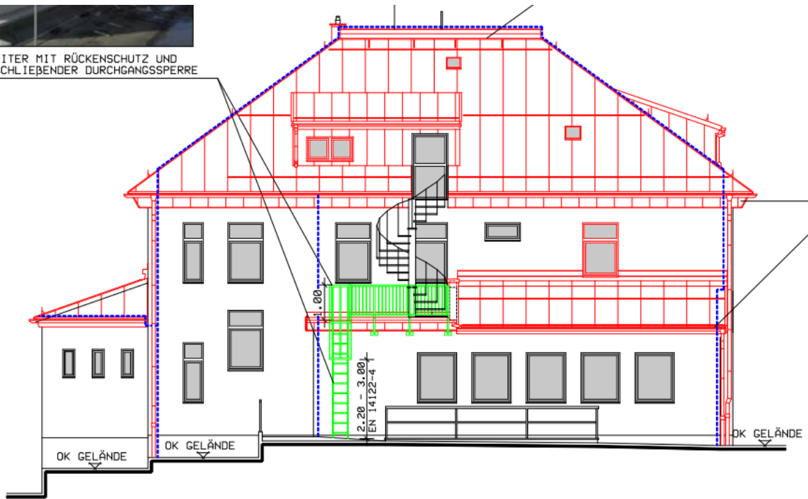
ANSICHT NORD
