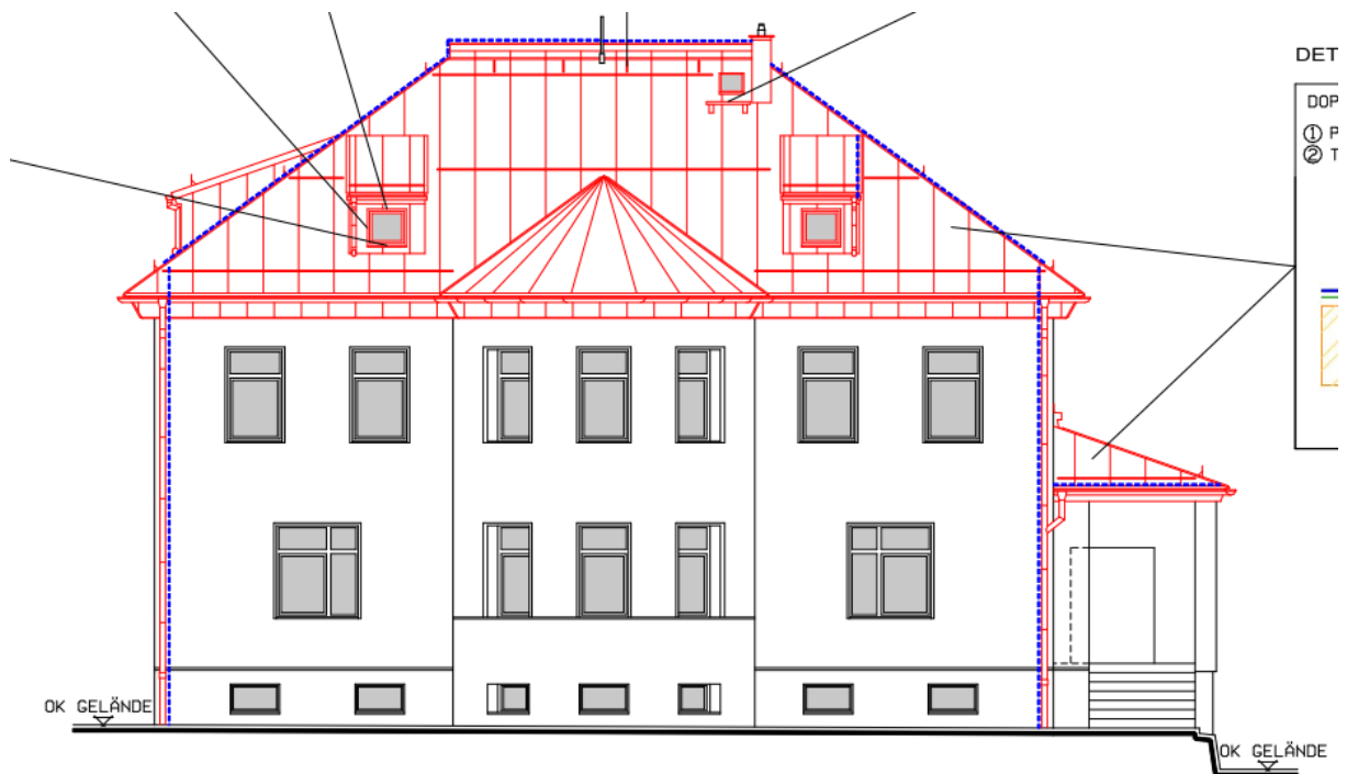
ANSICHT SÜD
