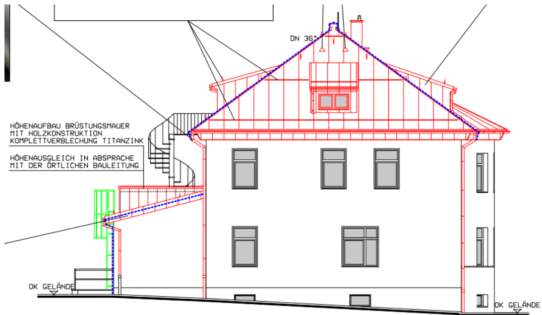
ANSICHT SÜD
