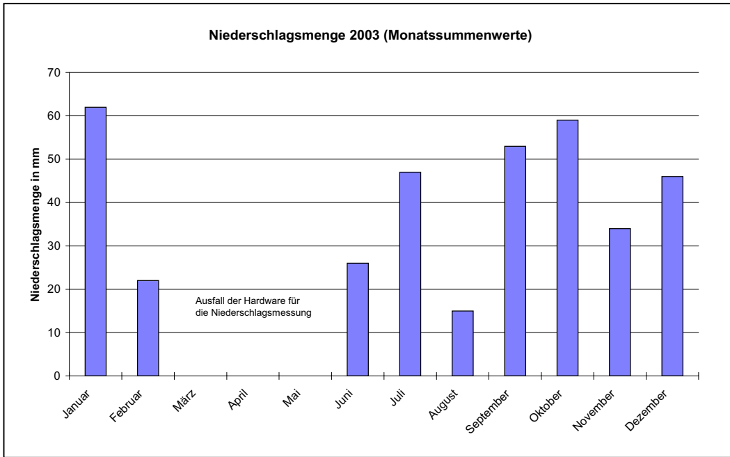
Diagramm 2: Aus dem Diagramm geht die Verteilung der Niederschläge auf die einzelnen Monate des Jahres hervor. In den Monaten März, April und Mai war durch einen Hardwaredefekt keine Erfassung der Niederschlagsmenge möglich.
